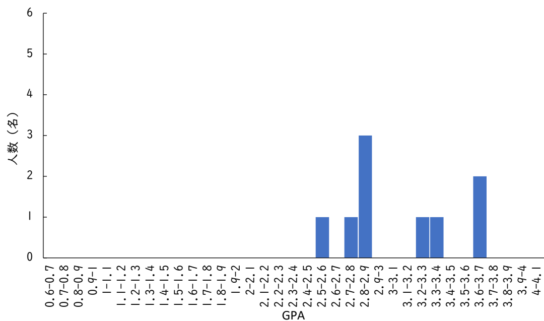
2年前期 GPA 度数分布
